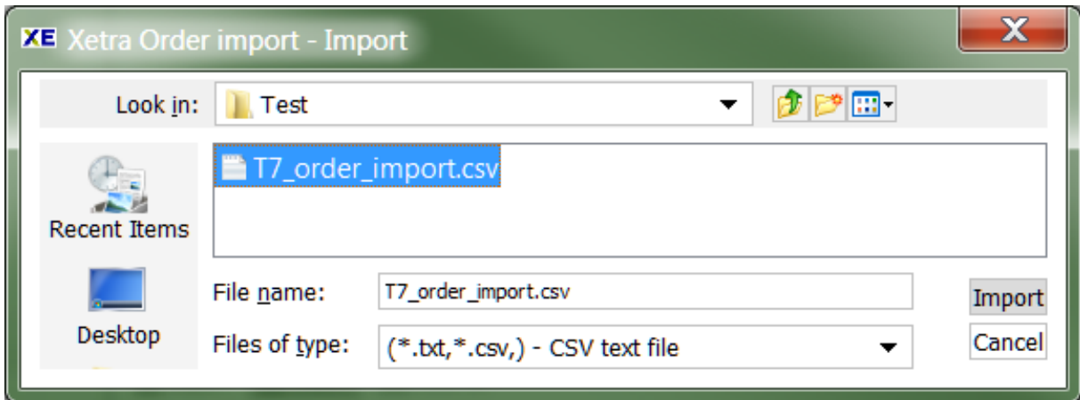
Fig. 30: Import Dialogue
