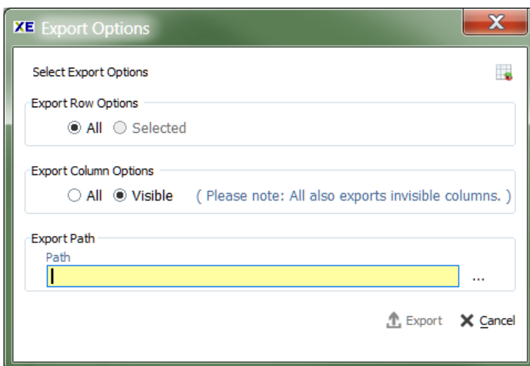
Fig. 31: Export Options
